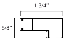
Traslape Puerta 69955
