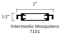
Horizontal Mosquitero 26533
