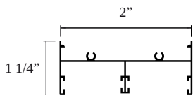
Jamba Cabezal 26534
