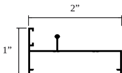
Riel Inferior 9953
