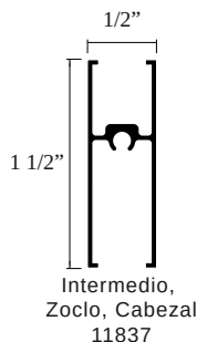
Zoclo Puerta 37825
