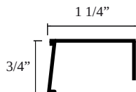
Junquillo 9112
