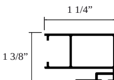
Traslape Ventana 37844
