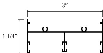
Jamba Cabezal 67826
