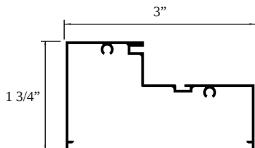
Escalonado 39136
