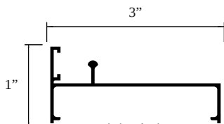
Riel Inferior 69957
