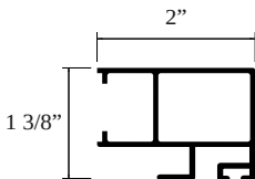
Traslape Puerta 67848
