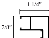
Traslape Ventana 39954
